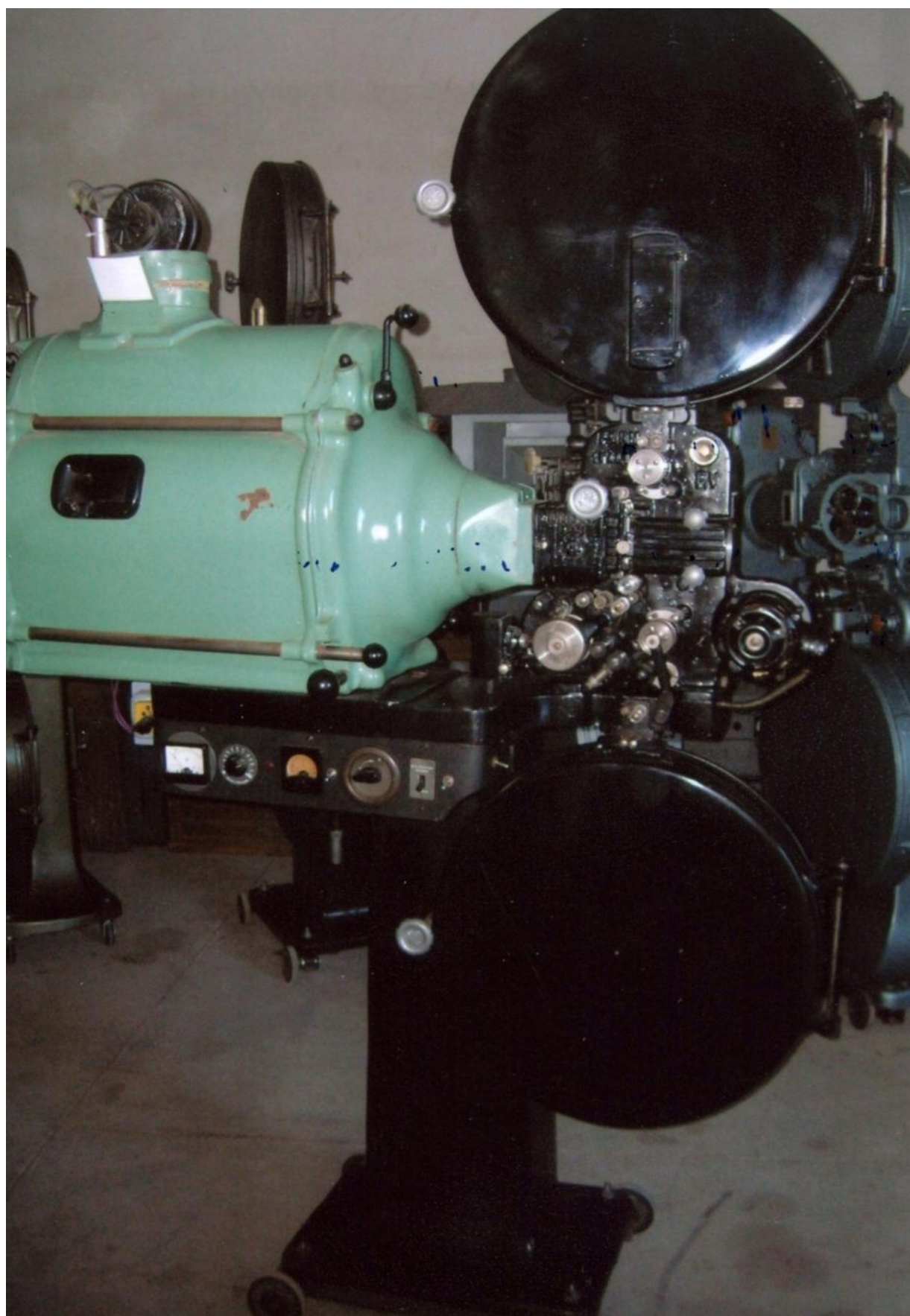
Fermini - Milano Modello: F.V. Sonoro: ottico Lampada: Arco "Microtecnica" Torino Anno: 1947
