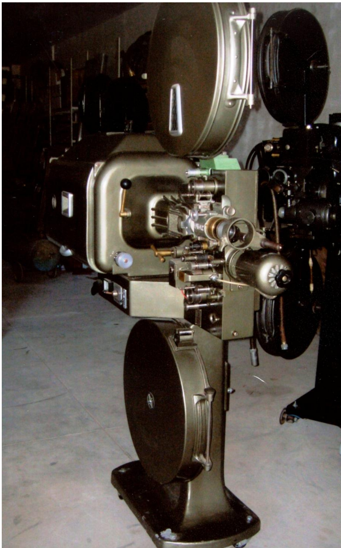
Pio Pion Modello: Super Silence
